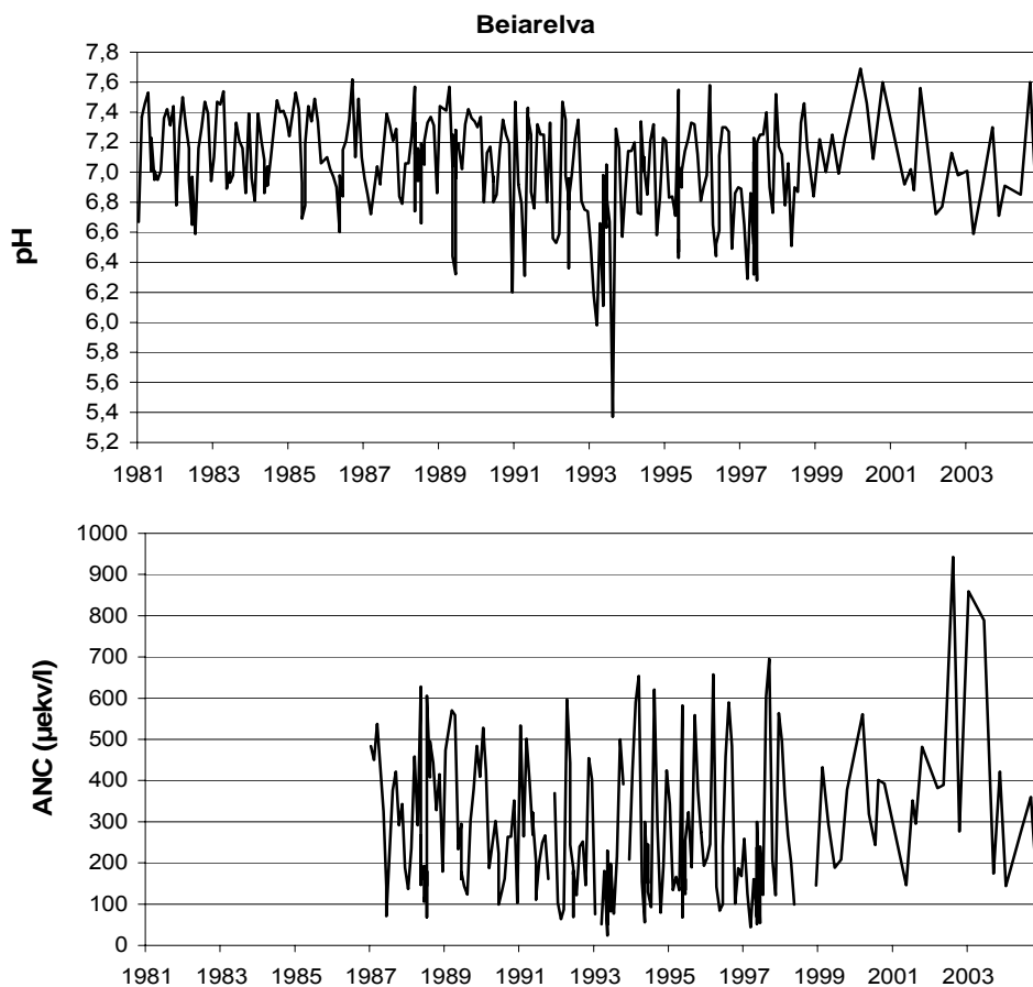
Figur 10. pH og ANC i Beiarelva i perioden 1981-2004.
