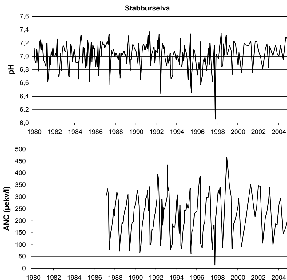
Figur 13. pH og ANC i Stabburselva i perioden 1980-2004.
