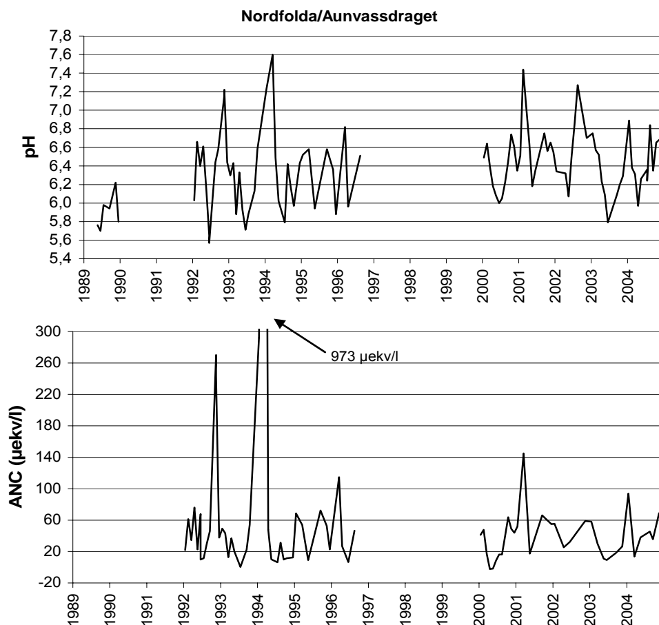
Figur 25. pH og ANC i Nordfolda i perioden 1989-2004. Data fra desember 2002 er tatt ut pga. usikker prøve kvalitet.
